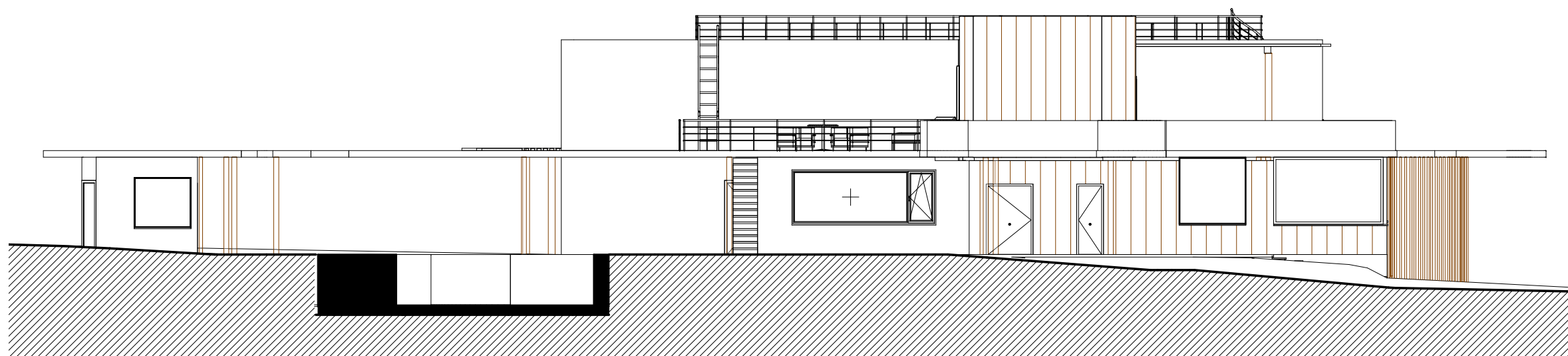
2 Alzado Sur e - 1:150
