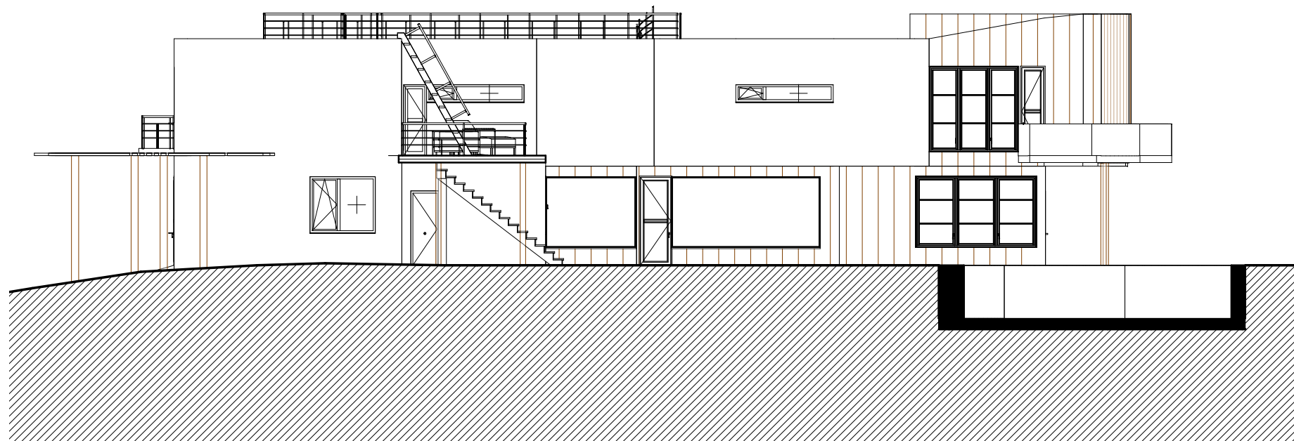
1 Alzado Oeste e - 1:150
