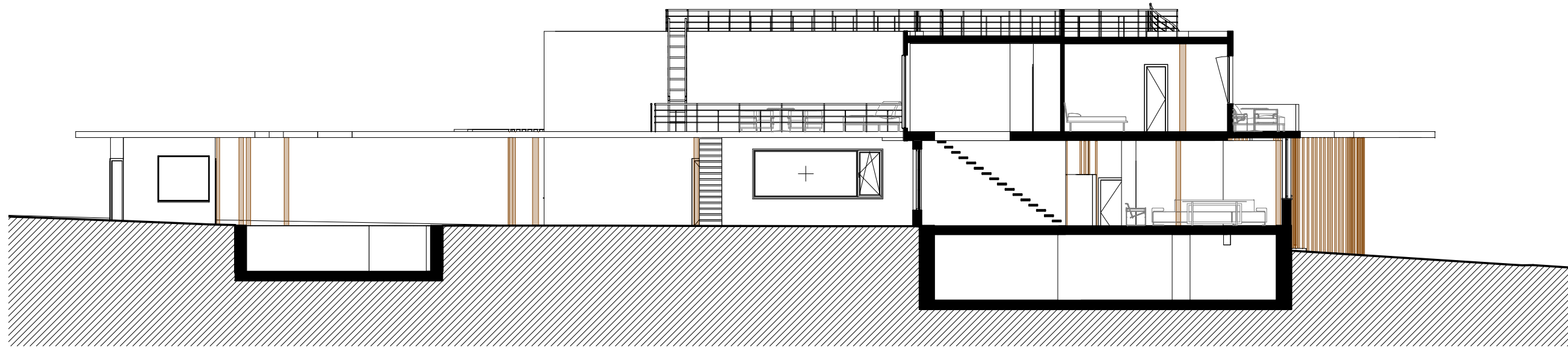
1 Sección Longitudinal 1 e - 1 : 150
