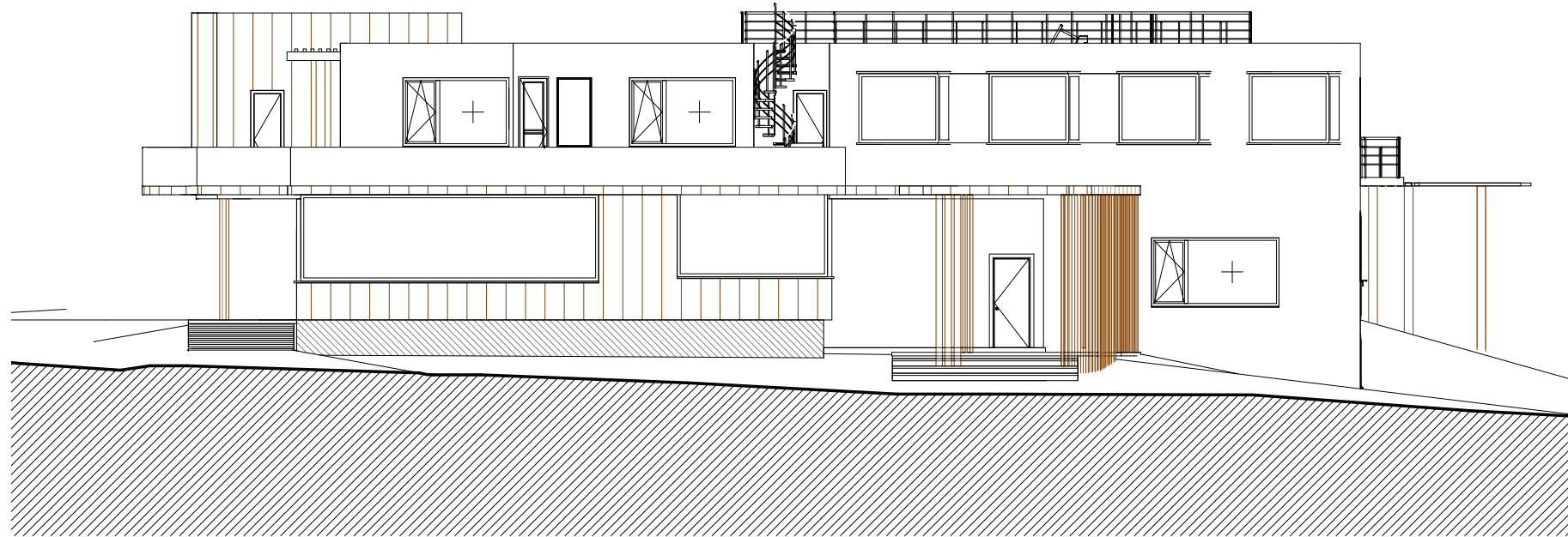
1 Alzado Este e - 1 : 150
