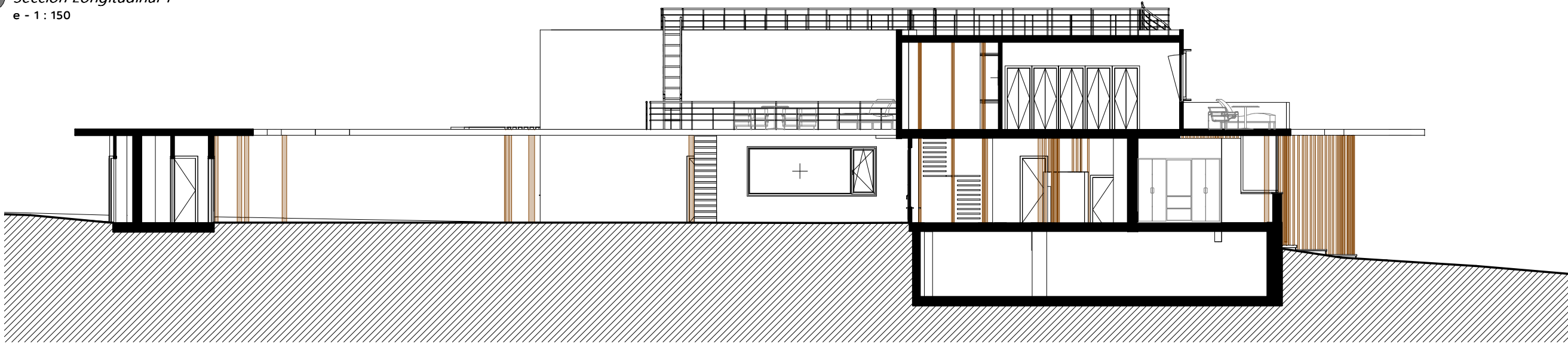
2 Sección Longitudinal 2 e - 1 : 150
