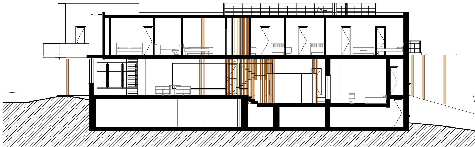
2 Sección Transversal B e - 1:150
