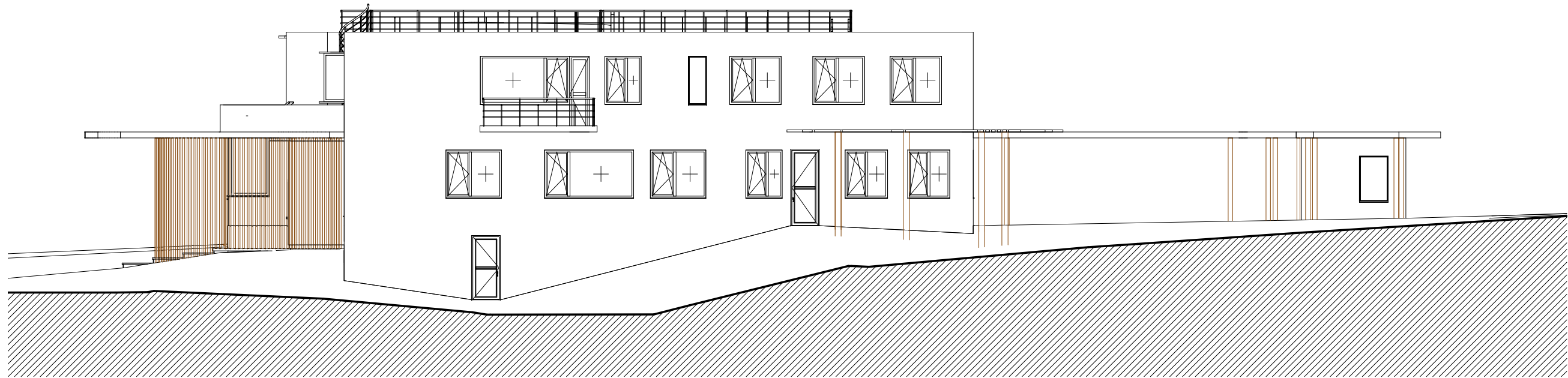
2 Alzado Norte e - 1 : 150
