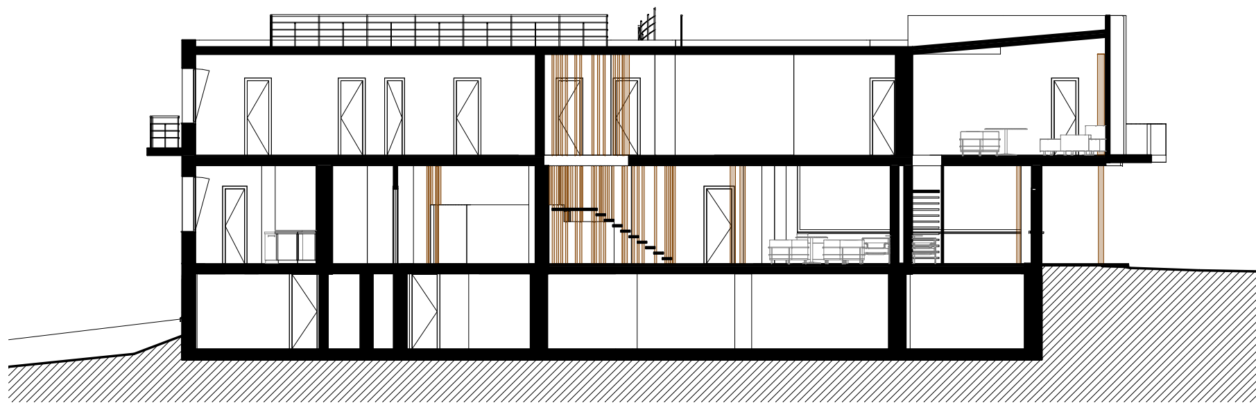
1 Sección Transversal A e - 1:150
